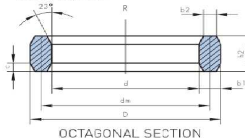
STYLE M18-RX
