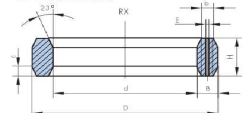
STYLE M18-RX
